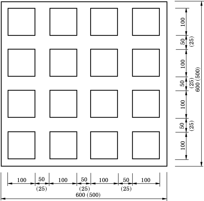
图 14 均布荷载聚氨酯块分布示意图
