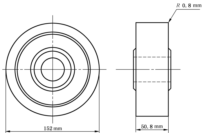
图 11 B 滚动轮尺寸示意图
