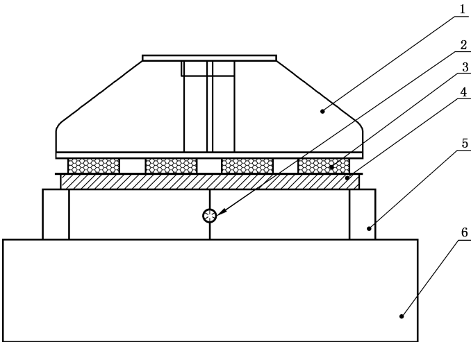
图 14 均布荷载聚氨酯块分布示意图
