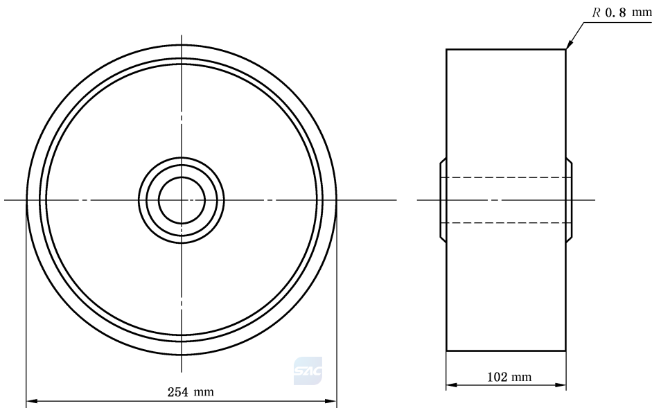
图 12 C 滚动轮尺寸示意图
